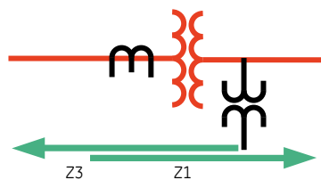
Z1 & Z3 looking through a transformer.
