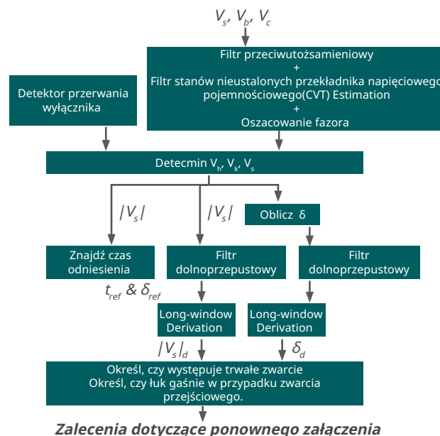
Rysunek 3: Adaptacyjne przetwarzanie logiki ponownego załączenia
