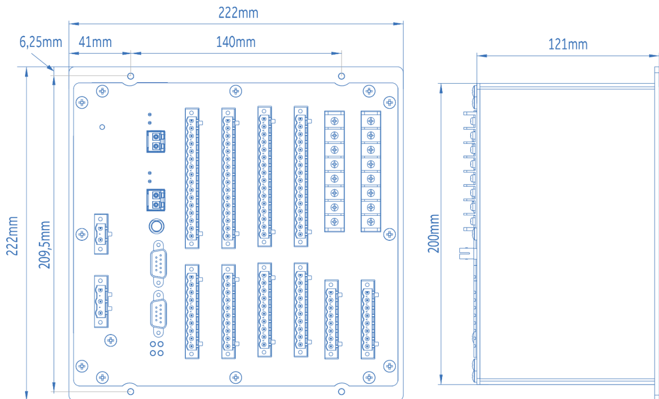
MU320E Dimensions
